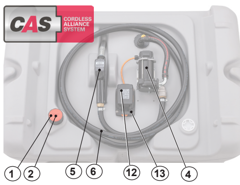
Pohled dovnitř zařízení DT-Mobil Easy 440 I
