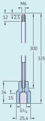
Verlängerungsrohr mit M6-Gewinde
